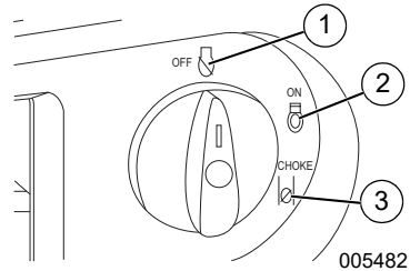
Figura 2-5. Interruptor (ejemplo)
