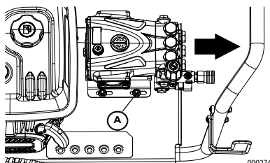
Figure 3-13. Éloignement de la pompe du moteur
