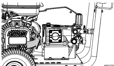
Figura 3-9. Vaciado de aceite de motor
